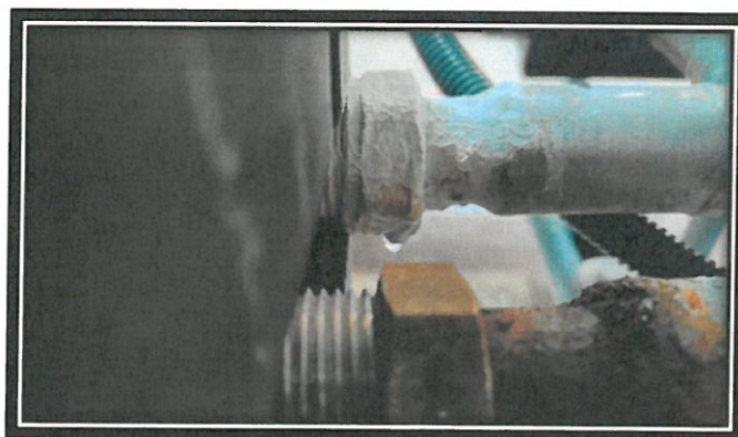
Wymiennik płytowy XB37-1 10L z widocznym wyciekem na śrubunku
