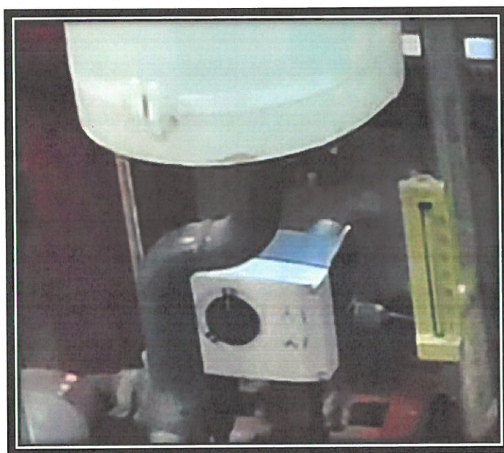
Głowica Zaworu regulacyjnego VM2 Dn 15
