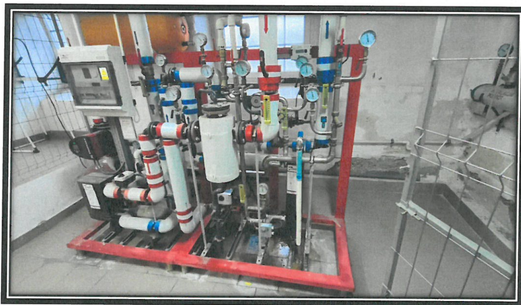
Węzeł kompaktowy dwufunkcyjny firmy Danfoss Sp. z o.o.
